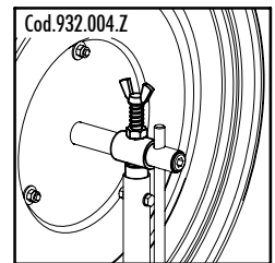
Frizione (optional) Clutch (optional)
