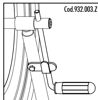
Bloccaggio rullo (optional) Reel stop (optional)
